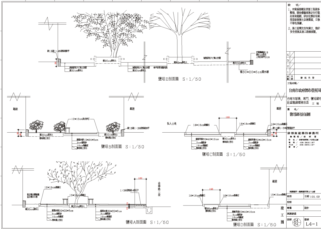
鹽埕國宅鄰棟綠帶剖面圖
